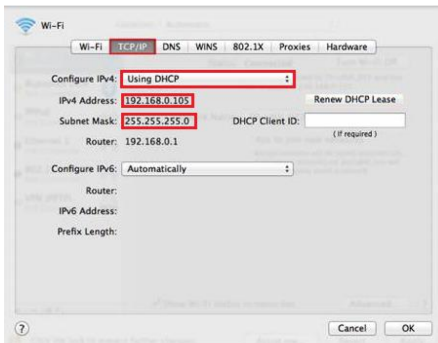
Figur 34: Ställ in nätverksinställningar
