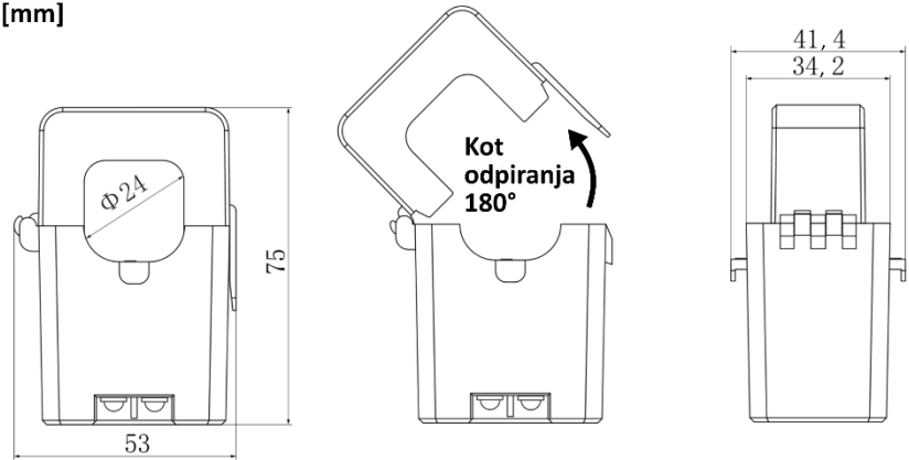
Slika 7: Dimenzije tokovnikov
