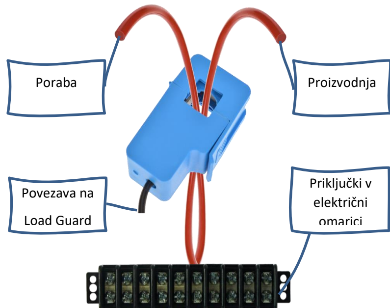
Slika 15: Tokovnik na dveh vodnikih
