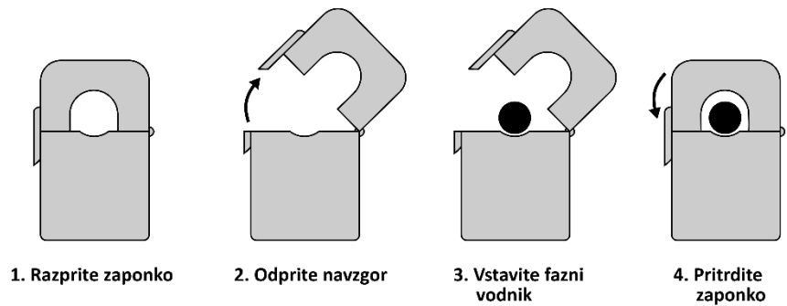
Slika 8: Povezovanje tokovnikov
